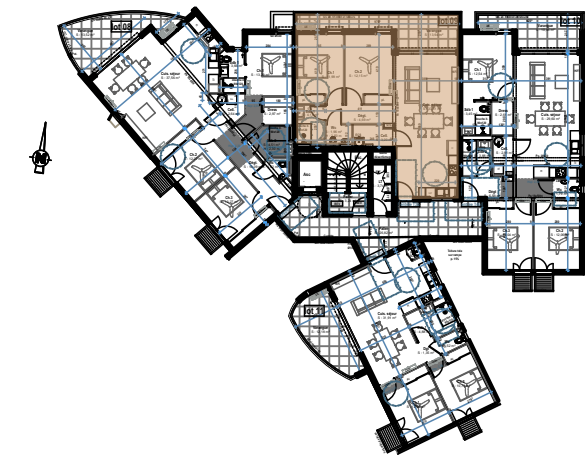
PLAN R+2
