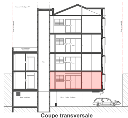
Coupe transversale
