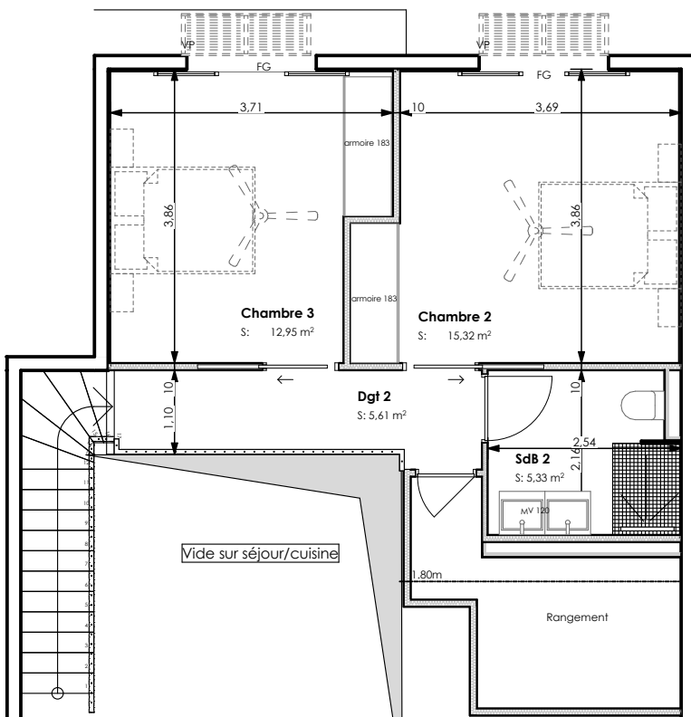
PLAN DU R + 2
