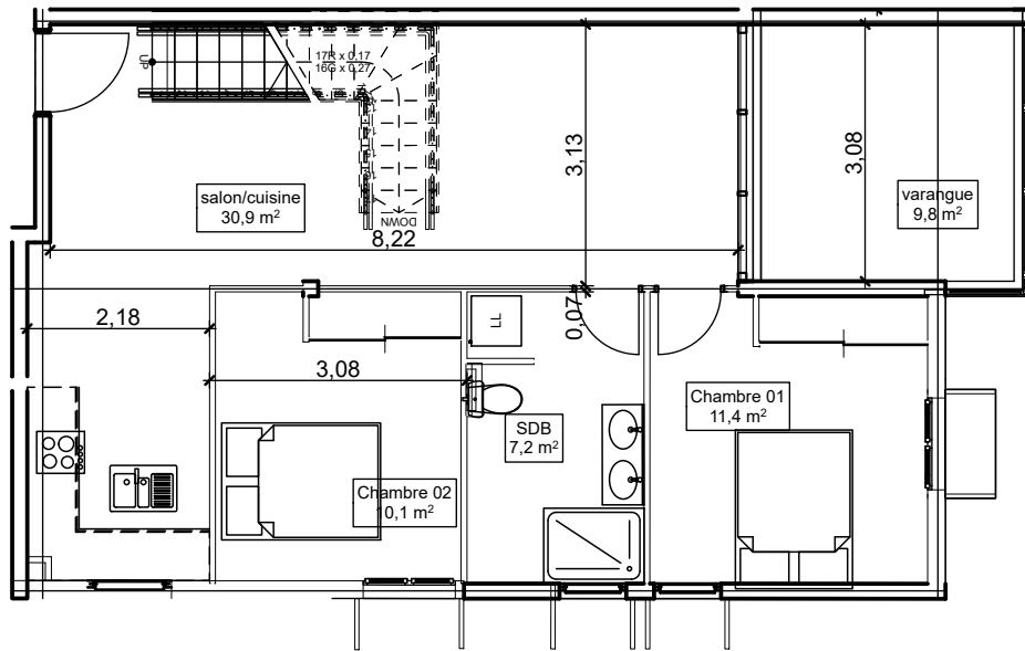
3. R+3 1:100
