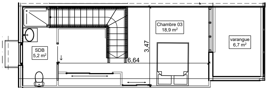
4. R+4 1:100
