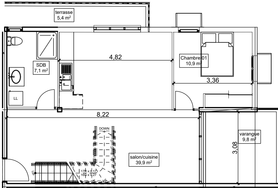
3. R+3 1:100
