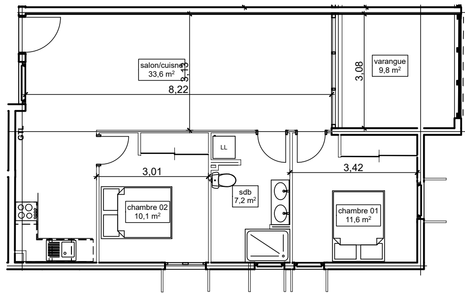
2. R+2 1:100
