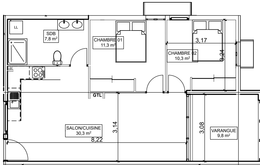
1. R+1 1:100
