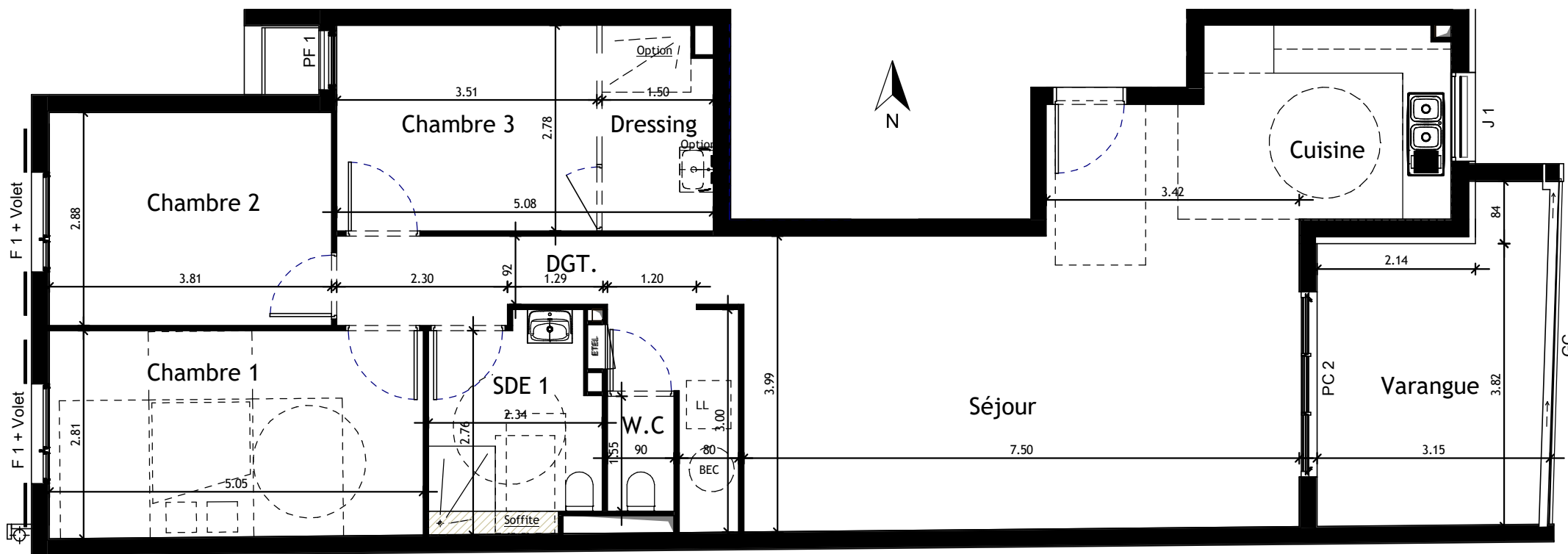
Logement N° 4
