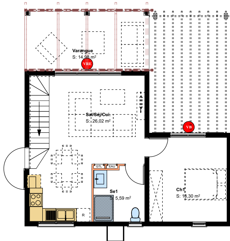
Rez de Chaussée
