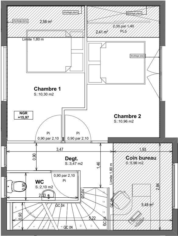
Niveau duplex
