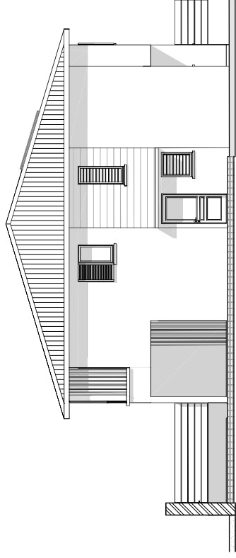
VILLA 1 -FACADE EST
