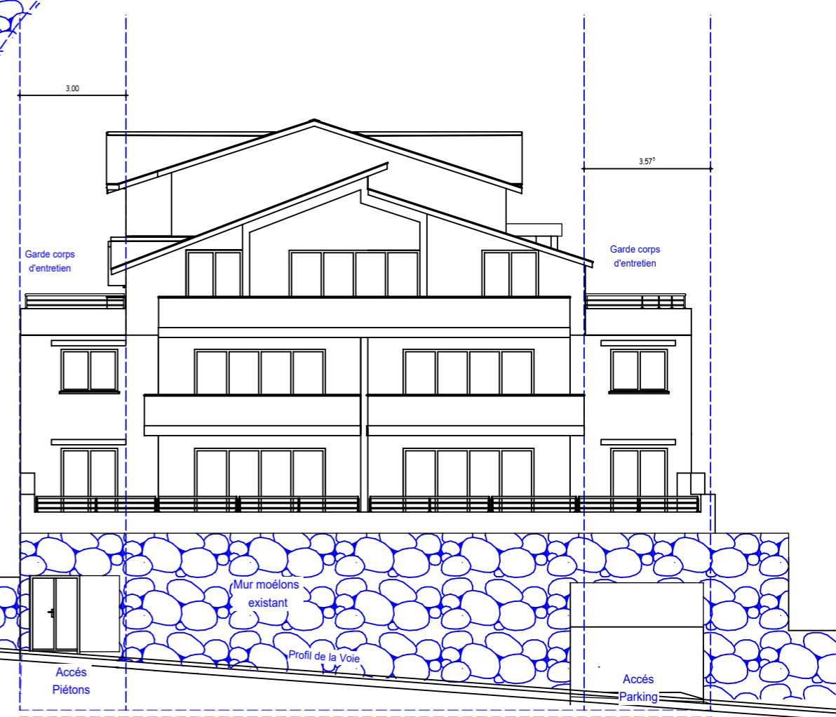
Façade OUEST
