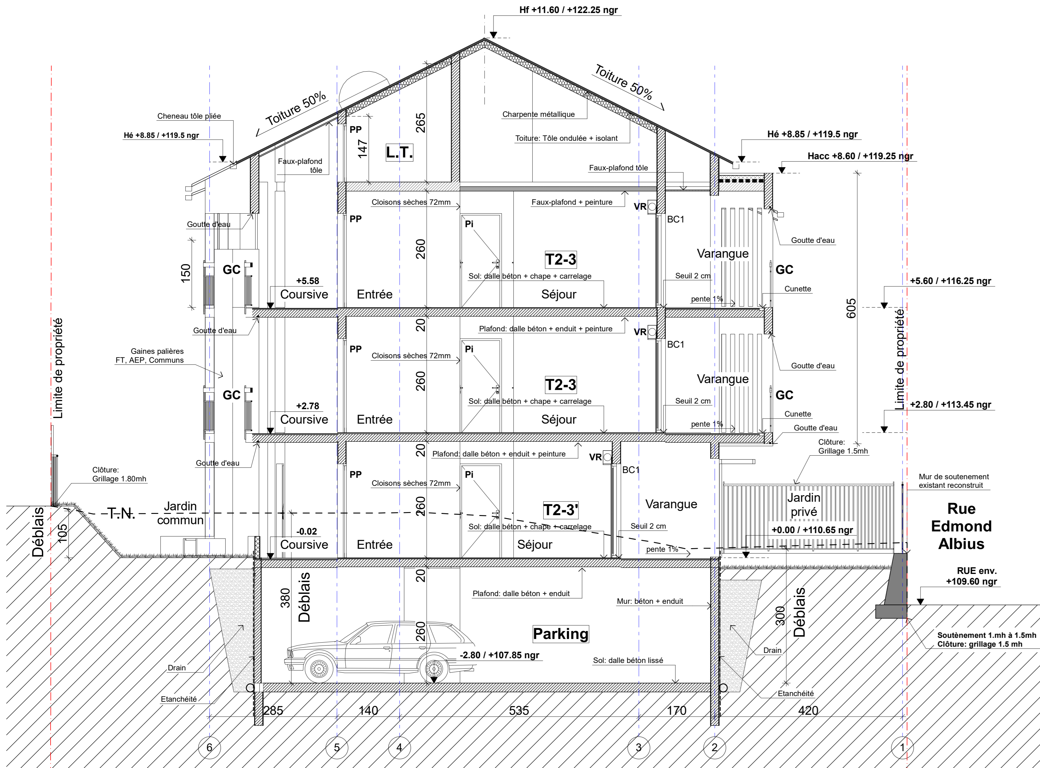
Coupe 5
