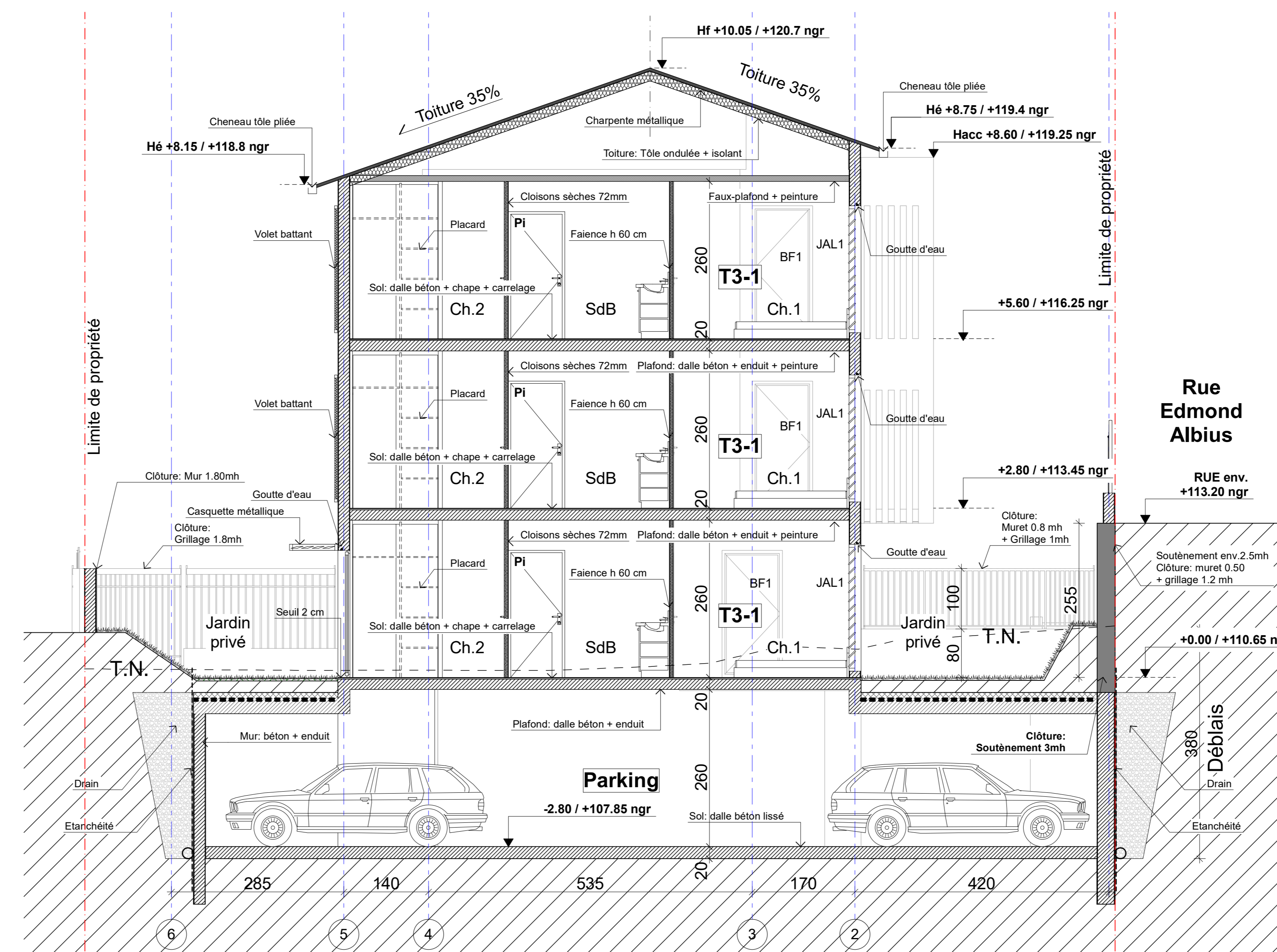
Coupe 8
