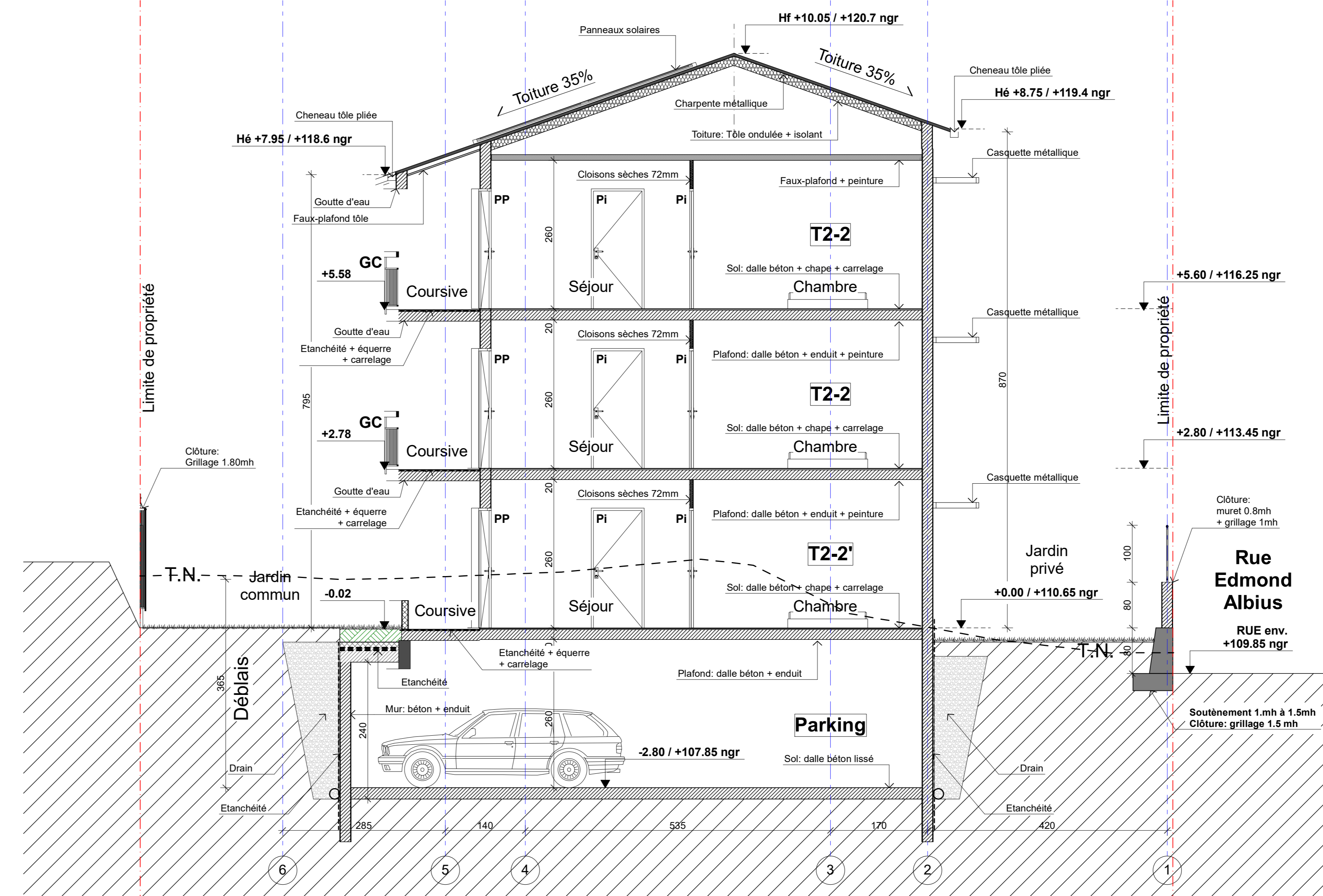
Coupe 6
