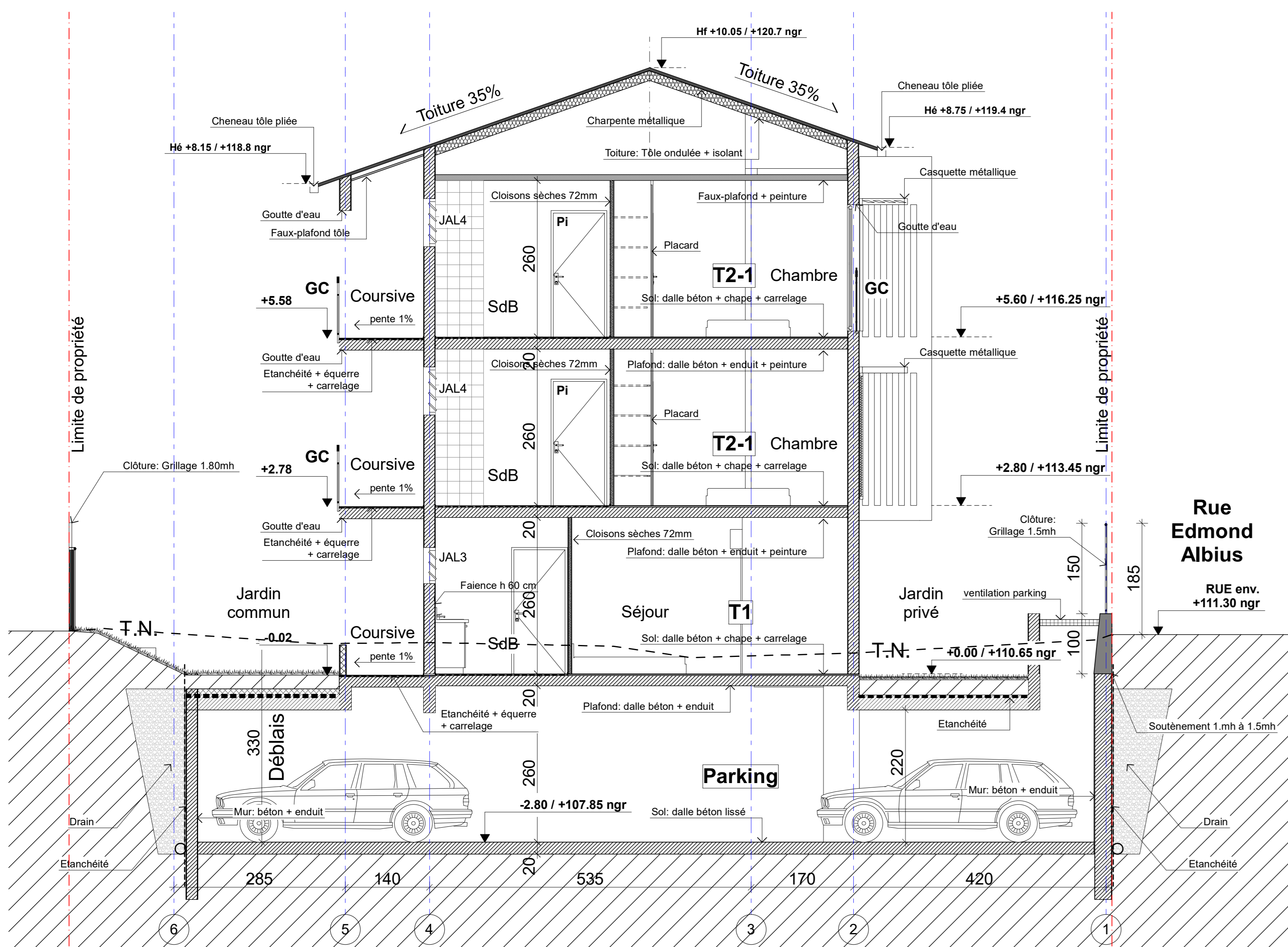
Coupe 7
