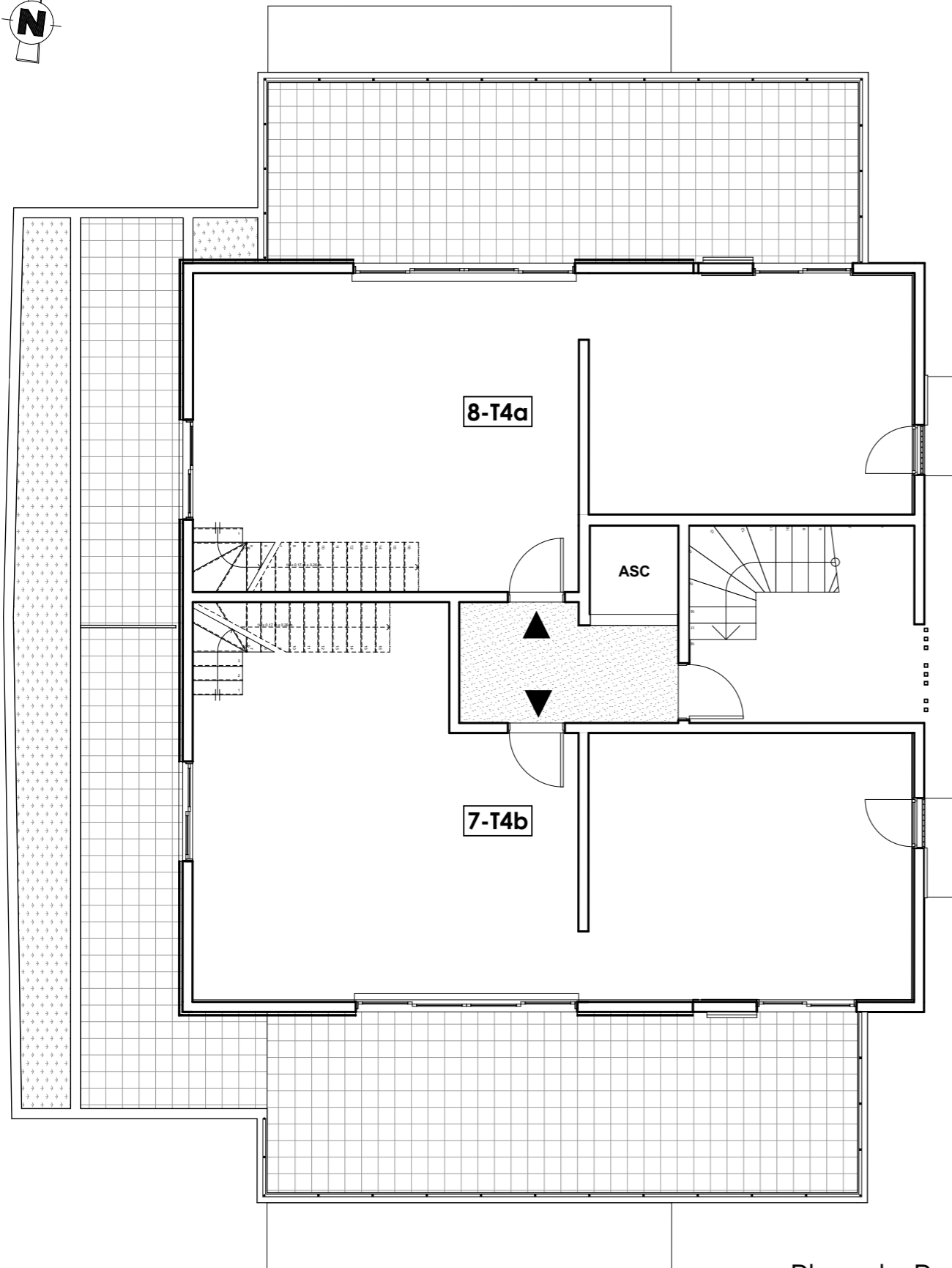
Plan du R+3
