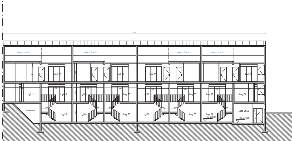
Coupe CC'
