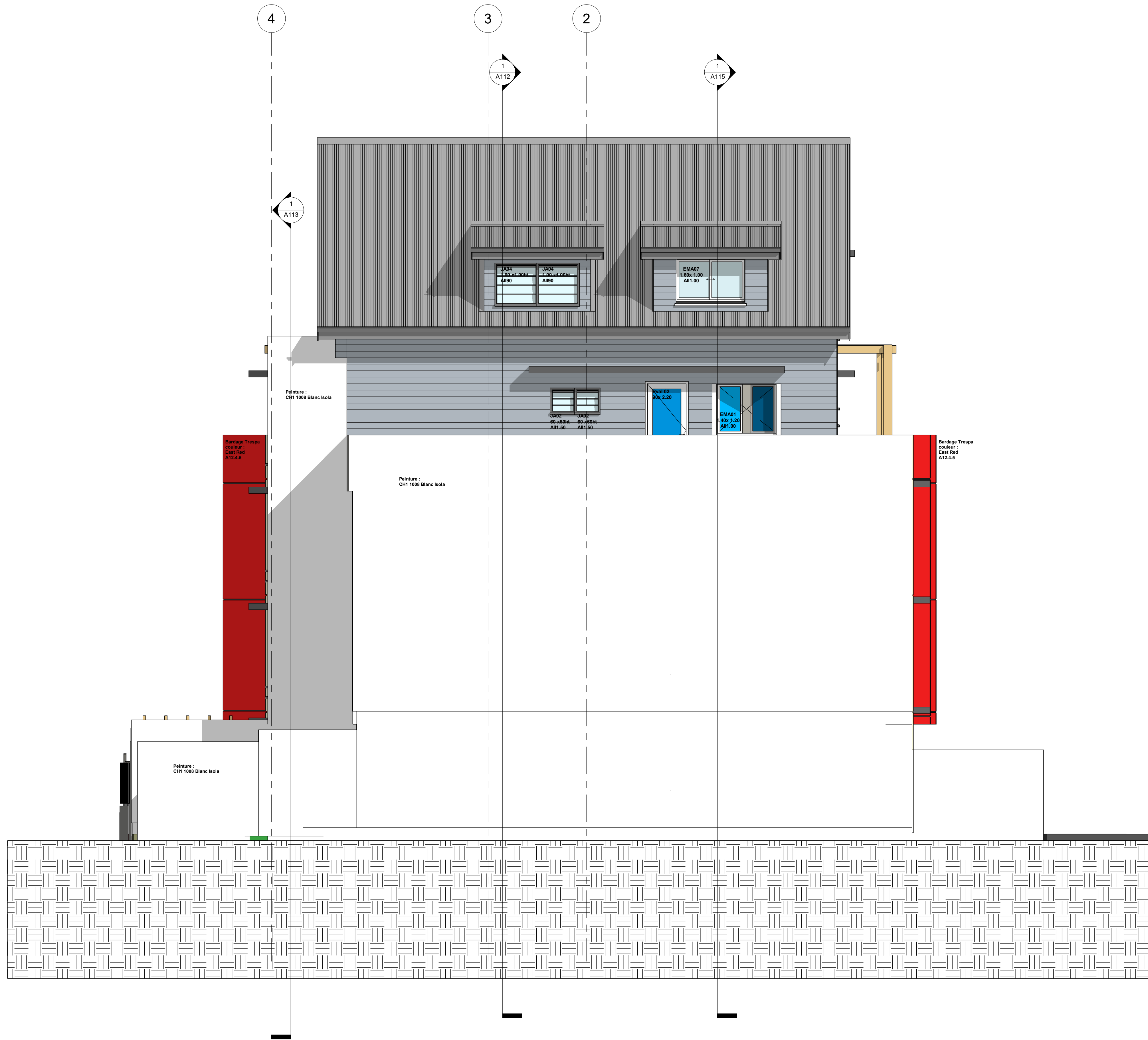
A109 Façade Arrière
