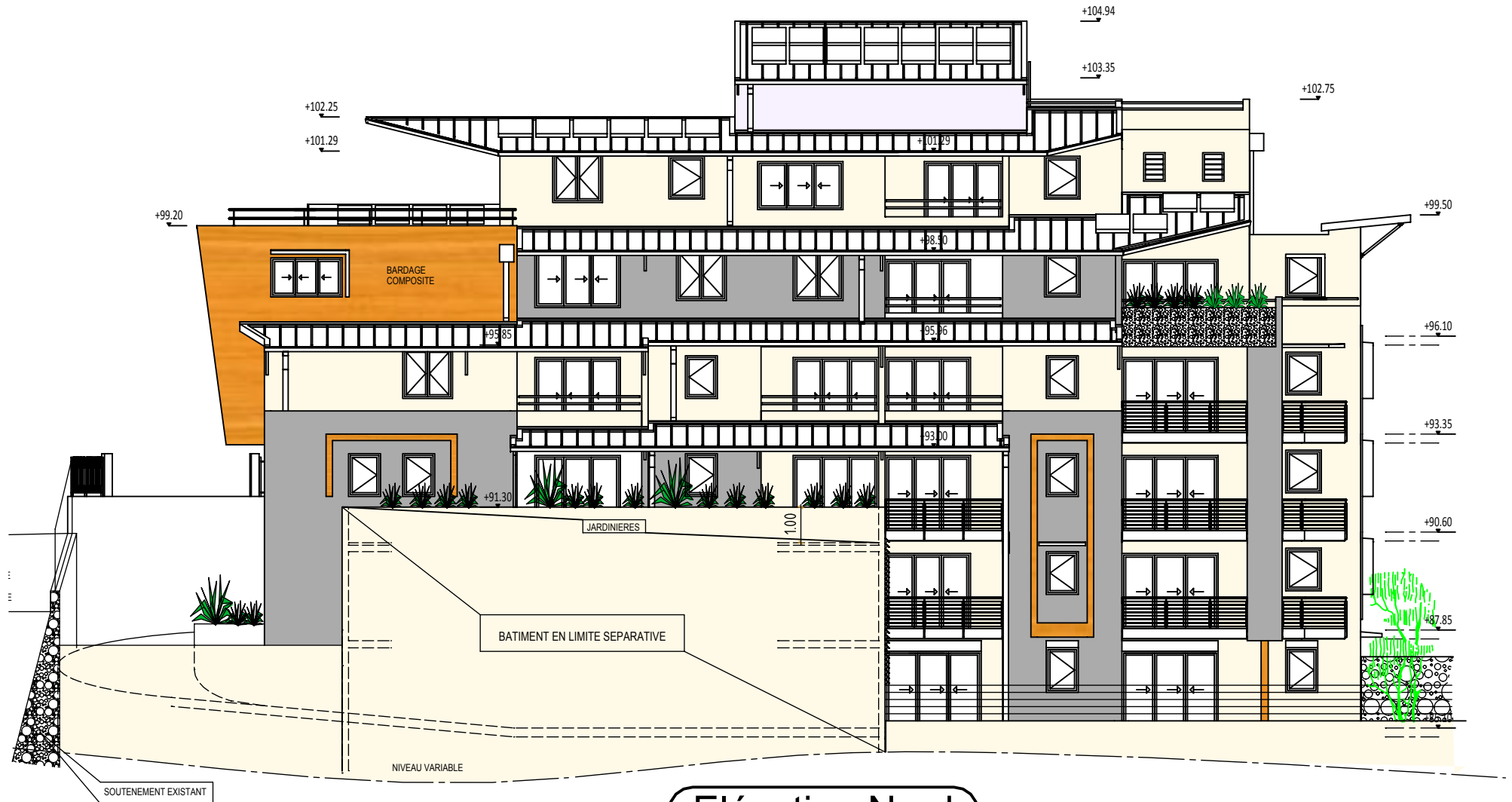
Elévation Nord
